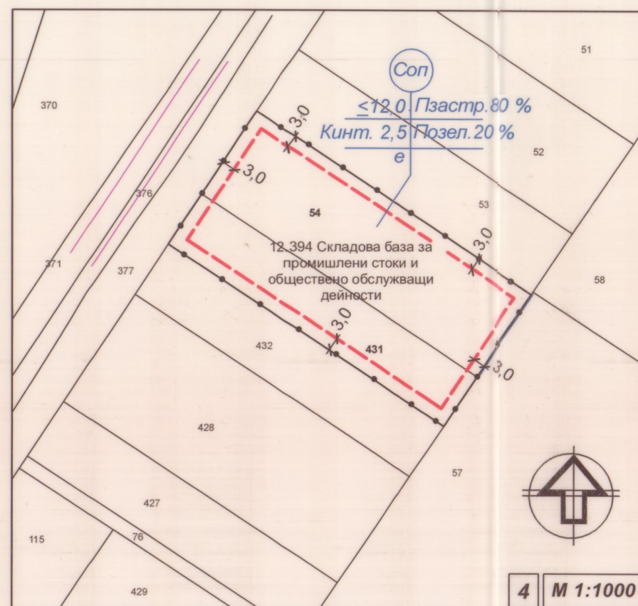
ПЛАН ЗА ЗАСТРОЯВАНЕ НА УПИ 12.394 СКЛАДОВА БАЗА ЗА ПРОМИШЛЕНИ СТОКИ И ОБЩЕСТВЕНО ОБСЛУЖВАЩИ ДЕЙНОСТИ, МЕСТНОСТ "БУНАР ЙОЛУ", ЗЕМЛИЩЕ НА ГР. КУКЛЕН, ОБЩИНА КУКЛЕН, ОБЛАСТ ПЛОВДИВ
